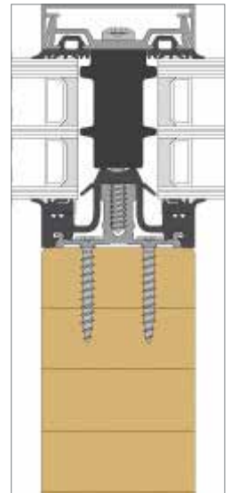
Modell-Zeichnung RAICO Therm+ H-I
